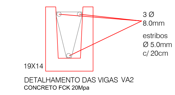
3 DETALHES Esc. 1:75
